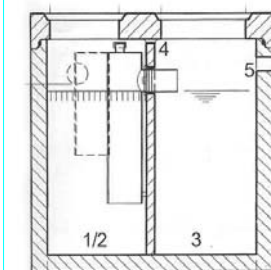
SX9 installation d'électro-séparation
